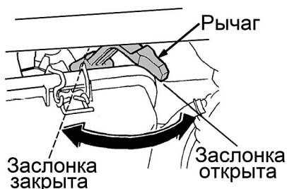
Рис. 10 Рычаг управления воздушной заслонкой IGG3600
