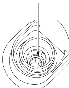
МАКСИМАЛЬНЫЙ УРОВЕНЬ ТОПЛИВА
