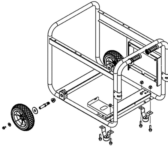
Рис. 4 Установка транспортировочных колес и опор рамы
